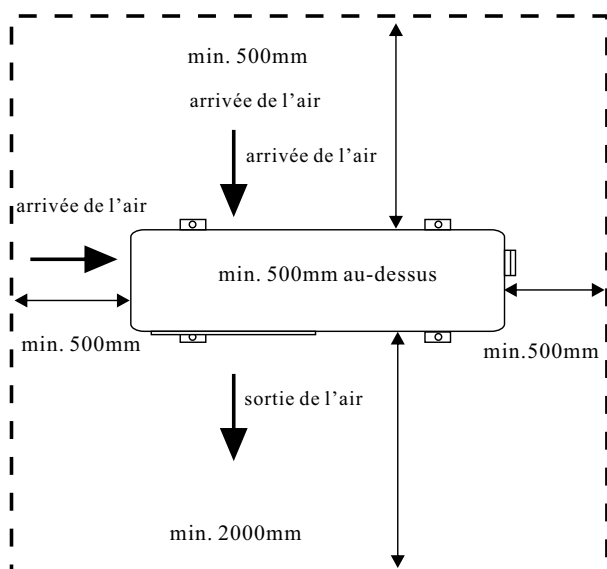
Modèle avec évacuation horizontale
